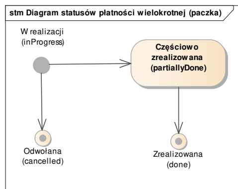
Diagram 9. Statusy płatności wielokrotnej (paczka przelewów)
